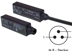
M 8 - Stecker
