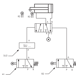
Zylinder 2
