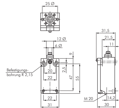
Kuppenstößel
