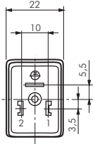
Typ CO 15-M-24V=
