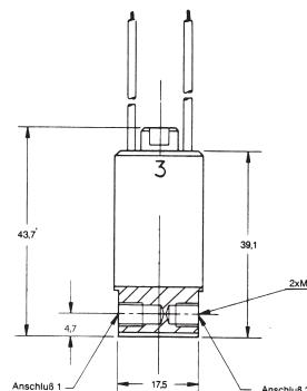
Typ M 2M5 ES..
