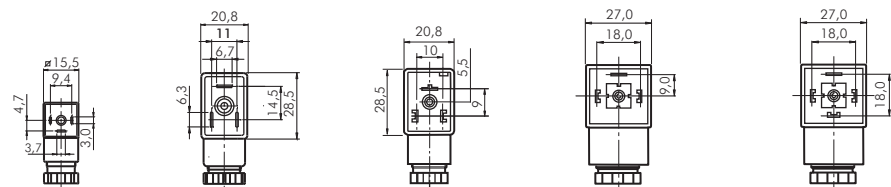
Größe 0 (Typ ST 00) (Industriennorm C) Größe 1 (Typ ST 01) (Industriennorm B) Größe 1 (Typ ST 01 DIN B) (DIN/EN-B) Größe 3 (Typ ST 03) (DIN/EN-A) Größe 3 (Typ ST 04) (DIN/EN-A)
