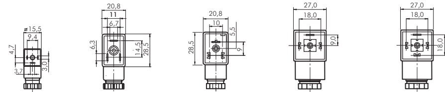
Größe 0 (Typ ST 00) (Industrienorm C)
