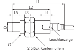
Typ mit Kabel, nicht bündig einbaubar
