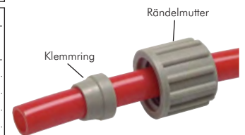
Anschlussprinzip „1“
