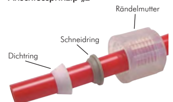
Anschlussprinzip „2“
