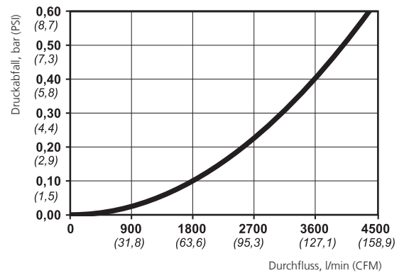
LUFTDURCHSATZ
