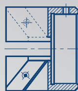
Rohrfräser 30° ID 16 - AD 50 mm Art. 091501101
