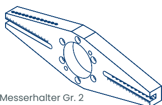
Messerhalter ID 280 - AD 711 mm Art. 091503168
