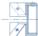
Rohrfräser 30° ID 11 - AD 22 mm Art. 091505348
