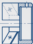
Rohrfräser 30° ID 25 - AD 58 mm Art. 091501102
