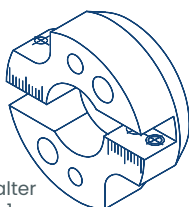
Rohrfräser 30° ID 11 - AD 22 mm Art. 091505348
